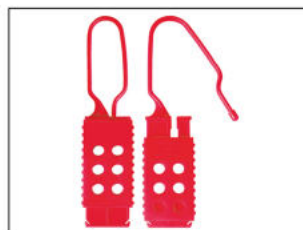
LU428 - Plastica per applicazioni elettriche, apertura 25x63 mm., per 6 lucchetti
